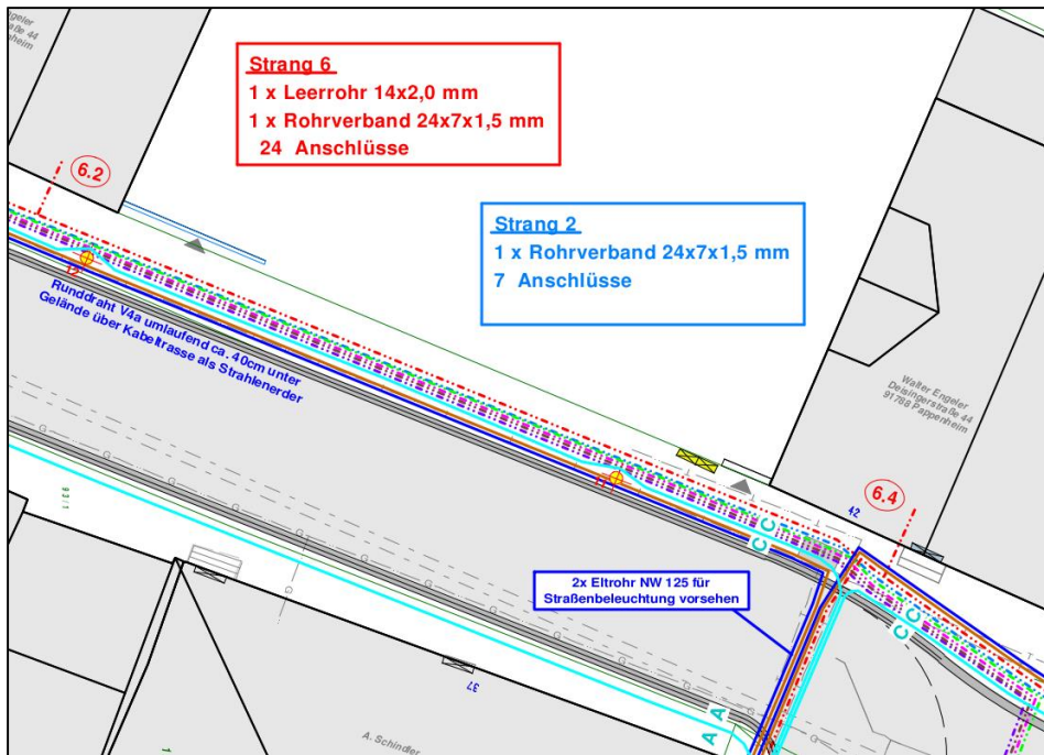
Ausschnitte aus den Verlegeplänen für Lichtwellenleiter
